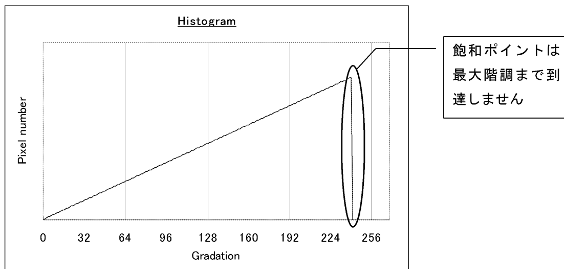
Fig 8.9.1. 階調補正機能例(8bit 出力)
