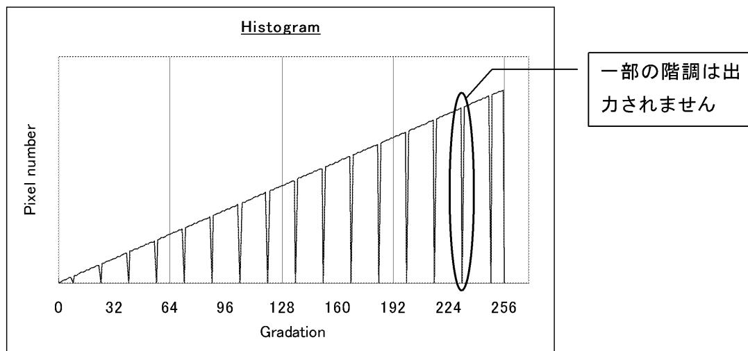
Fig 8.8. 本機の階調出力例(8bit 出力)
