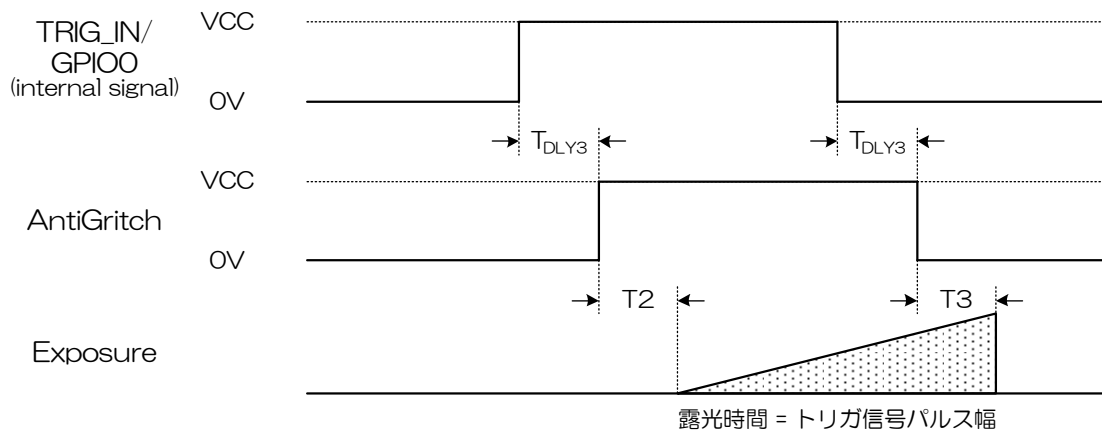
Pulse モード（全画素読み出し時）
