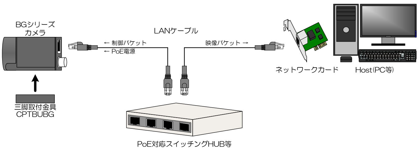
接続例
