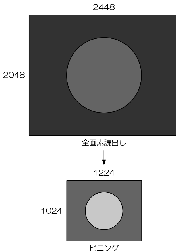
ビニング動作のイメージ (BG505LMG, 2x2 ビニング)
