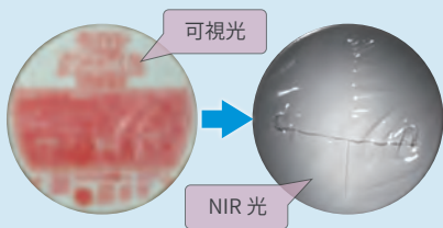
食品ラベル印刷の透過によるフィルム表面検査
