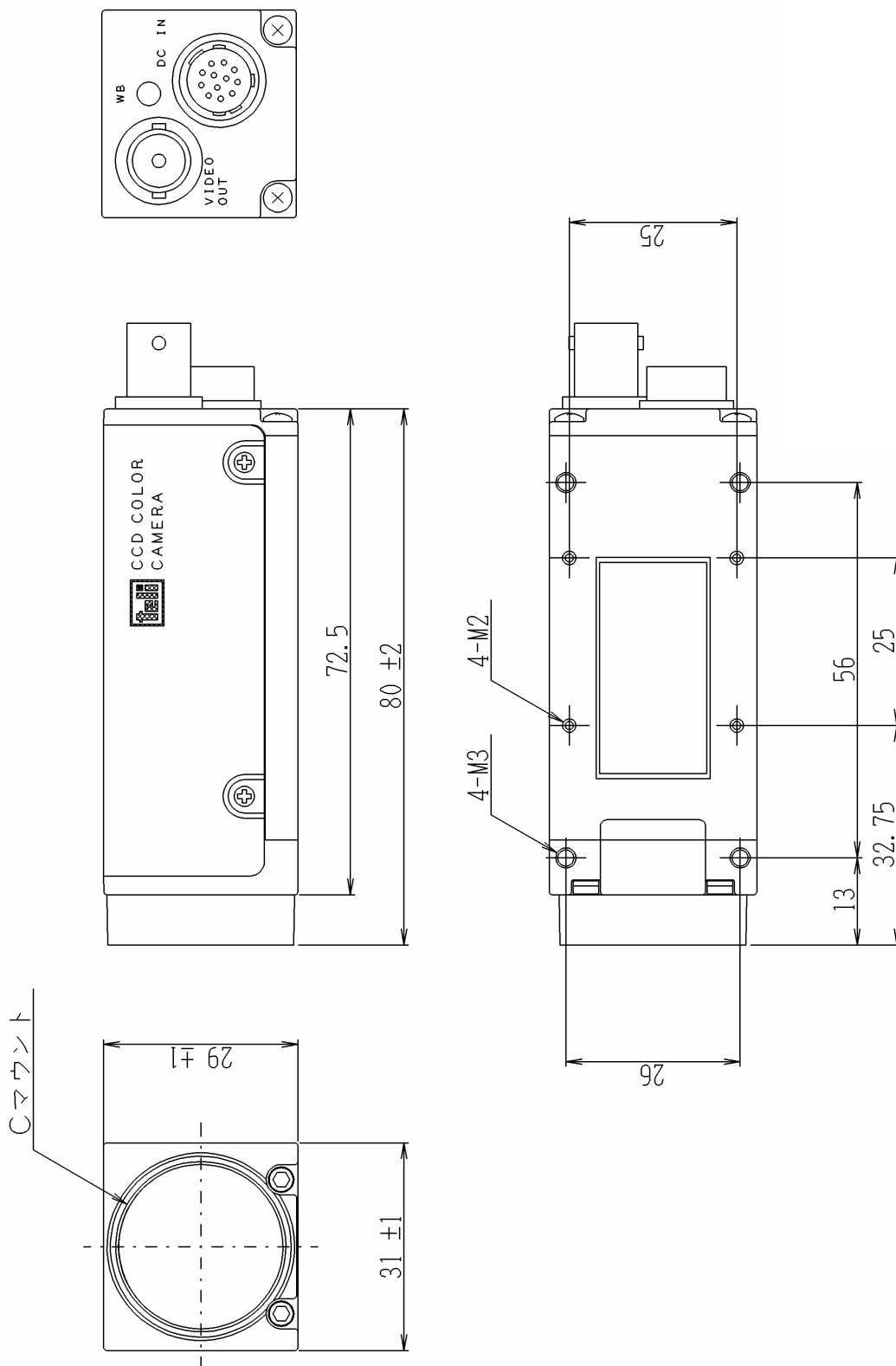
CS5260BD外形図
