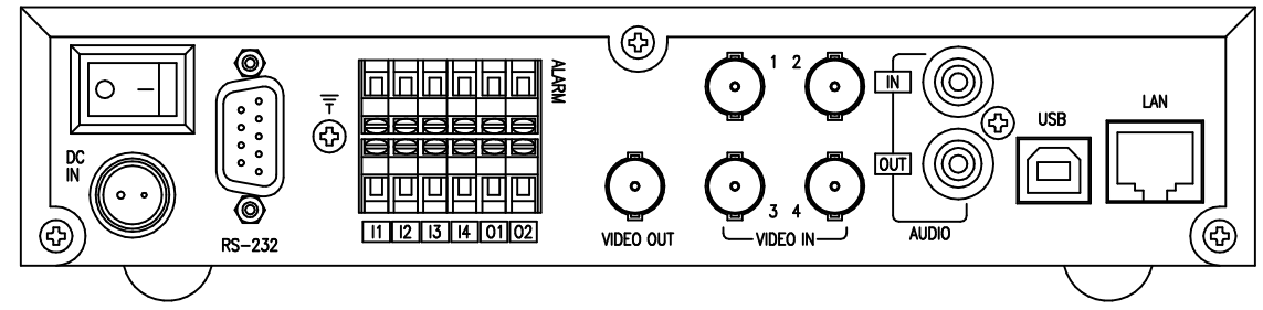
A矢視 背面図
