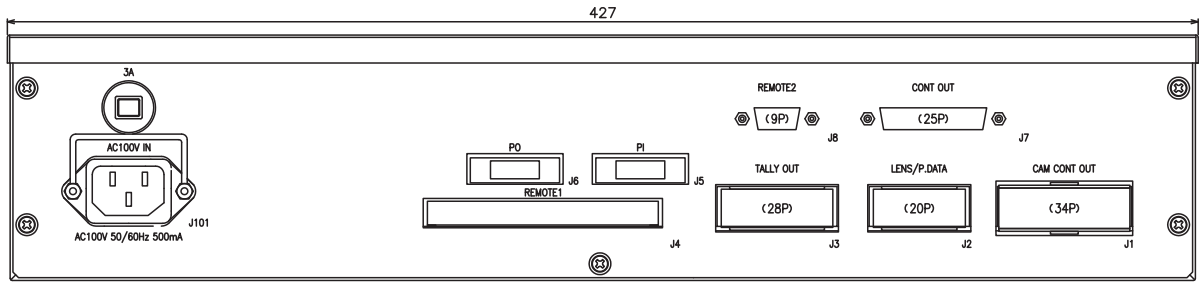
背面図
